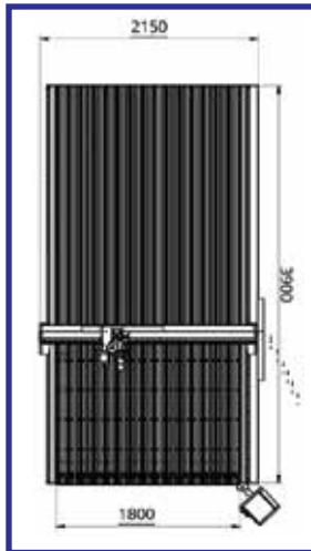
Optional Tufnol Vacuum Table
